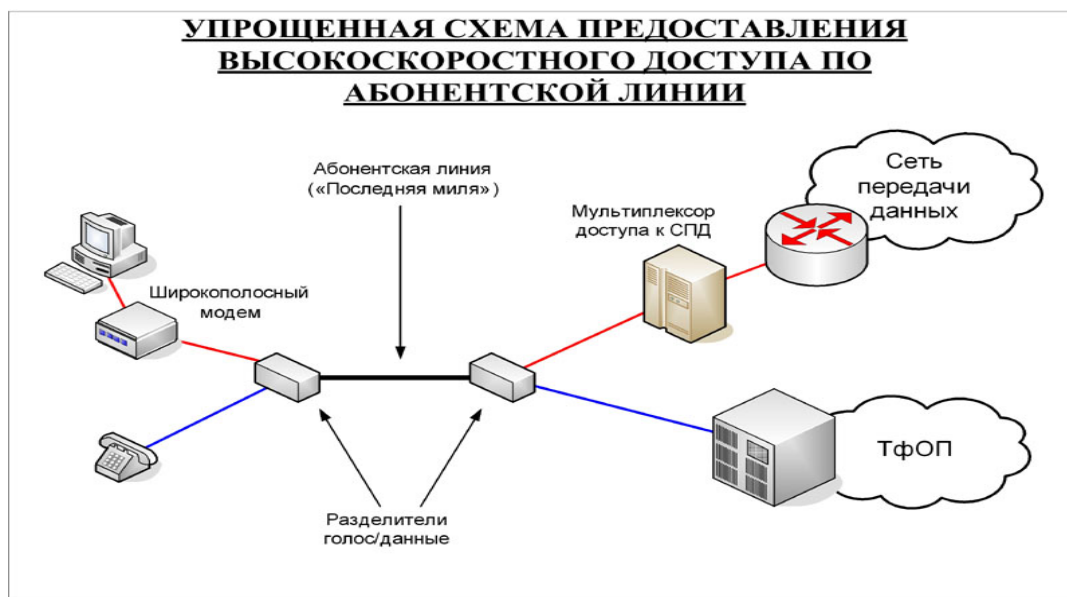
Рис.15: Схема организации цифрового абонентского доступа.
